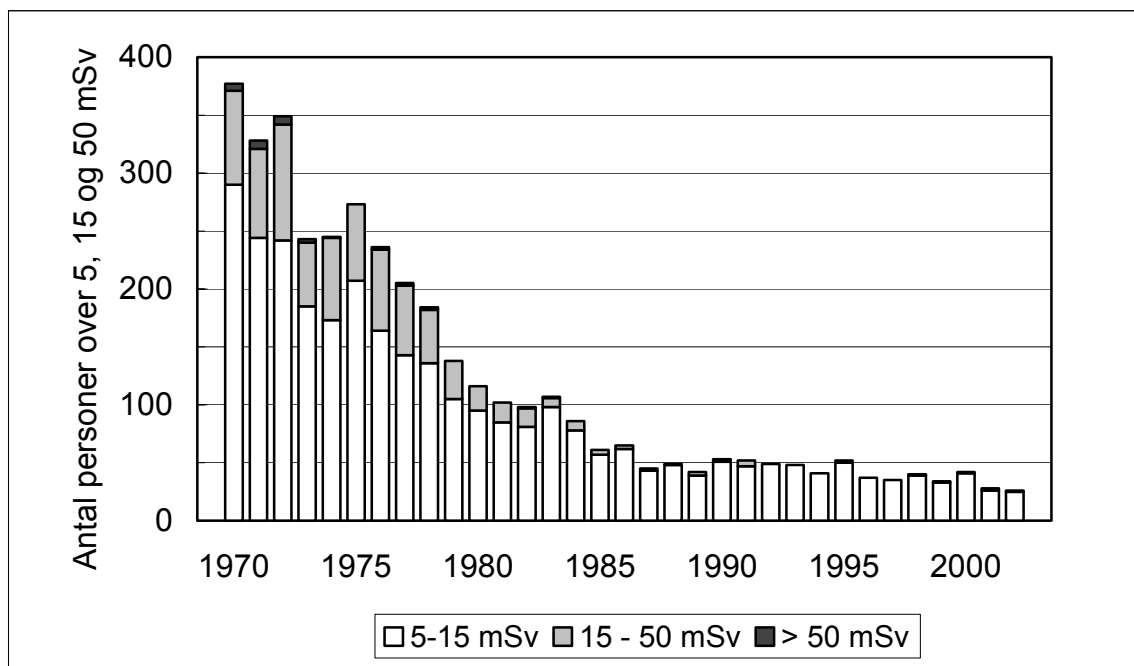
Fig. 2. Udviklingen i antallet af ”store doser” i perioden 1970 - 2002
