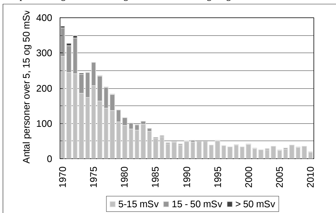
Figur 2. Udviklingen i antallet af "store doser" i perioden 1970 - 2010
